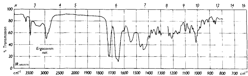
IR.-Spektren der synthetischen und natürlichen Alkaloide in \text{CH}_2\text{Cl}_2
